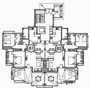
PLANTA BAJA
