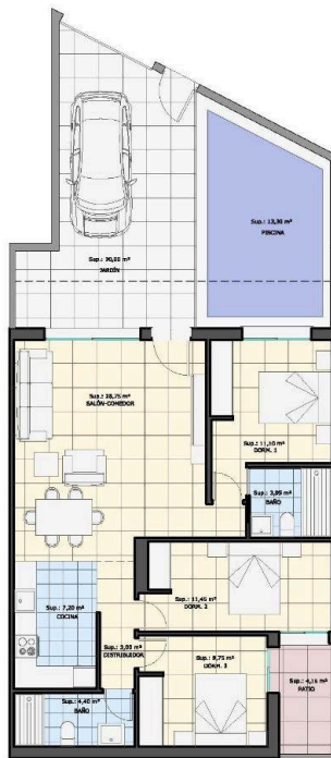
PLANTA BAJA
