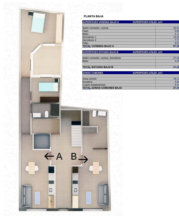
Planta Baja. Estudio B y Vivienda A
