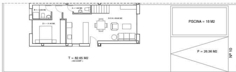
PLANTA BAJA
