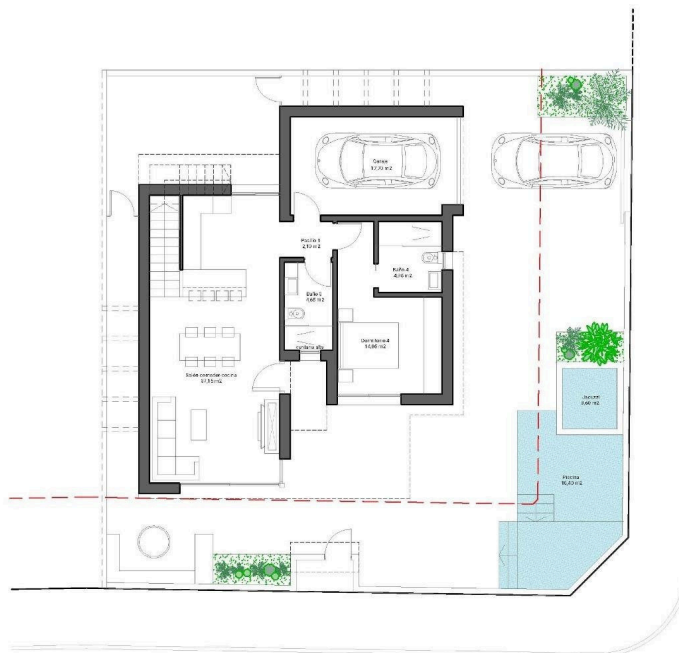
VILLA CON PISCINA EN SAN PEDRO DEL PINATAR OPCIÓN A.1.1. PLANTA BAJA.
