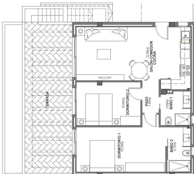
Planta Primera
