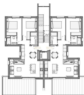
PLANTA PRIMERA
