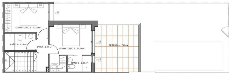
PLANTA PRIMERA
