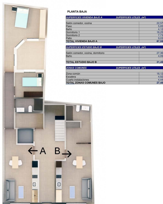
Planta Baja. Estudio B y Vivienda A
