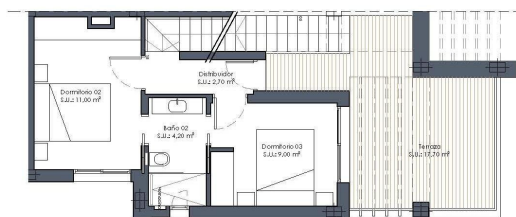
Planta primera
