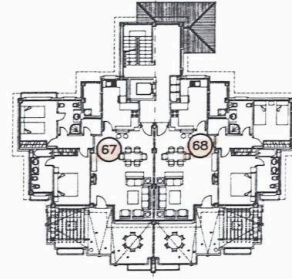
PLANTA TERCERA
